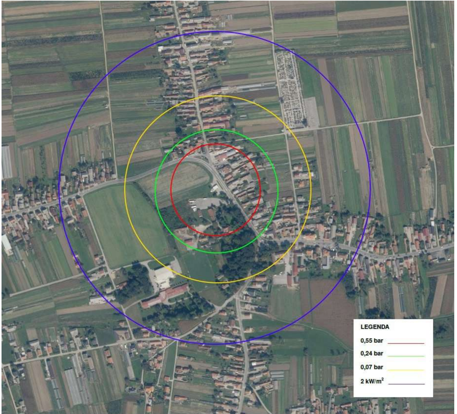
PRIKAZ MIKROLOKACIJE MPM VIDOVEC U SLUČAJU NAGOREG MOGUĆEG SLUČAJA EKSPLOZIJE CISTERNE GORIVA
